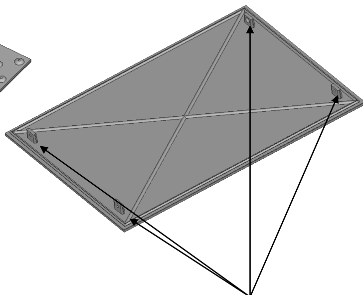
4 Pattes de scellement
