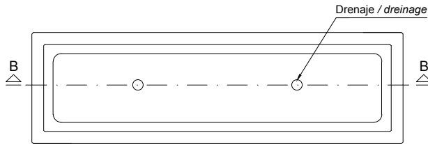
PLANTA / TOP VIEW
