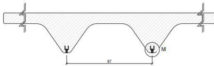
SECCIÓN A-A' / SECTION A-A'
