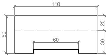
VUE DE PROFIL GAUCHE
