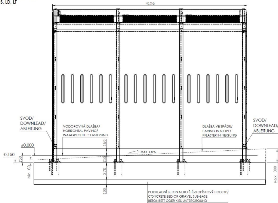
ŽÁKLADOVÁ DESKA / FOUNDATION BASEPLATE / FUNDAMENTPLATTE KUBATURA BETONU / CONCRETE CUBATURE / BETONRAUMINHALT - 3.70m3
