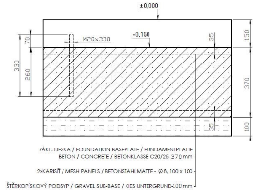
ŽÁKLADOVÁ DESKA / FOUNDATION BASEPLATE / FUNDAMENTPLATTE 5000x2000x370 mm
