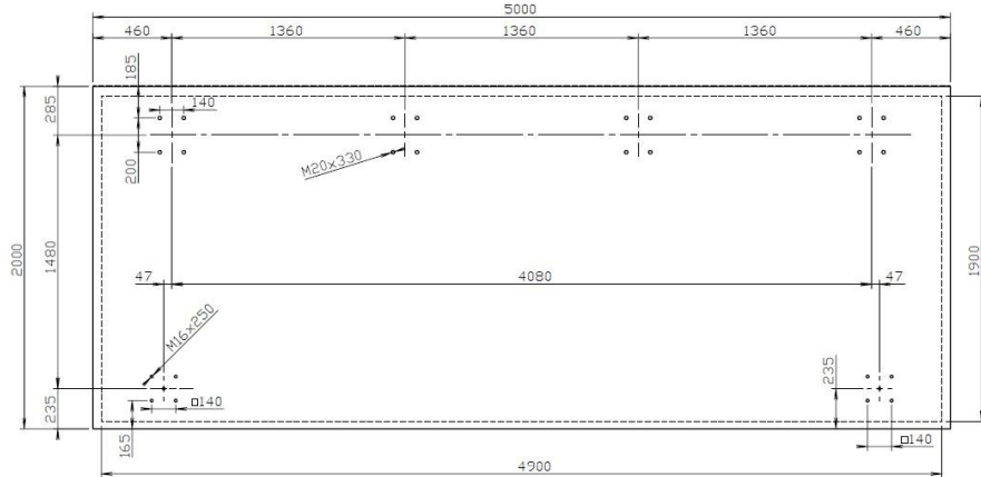
ŽÁKLADOVÁ DESKA / FOUNDATION BASEPLATE / FUNDAMENTPLATTE KUBATURA BETONU / CONCRETE CUBATURE / BETONRAUMINHALT - 3.70m3
