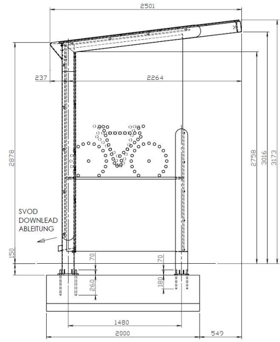
ŽÁKLADOVÁ DESKA / FOUNDATION BASEPLATE / FUNDAMENTPLATTE 5000x2000x370 mm
