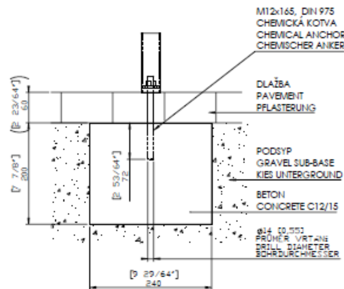
DETAIL B 1 : 5
